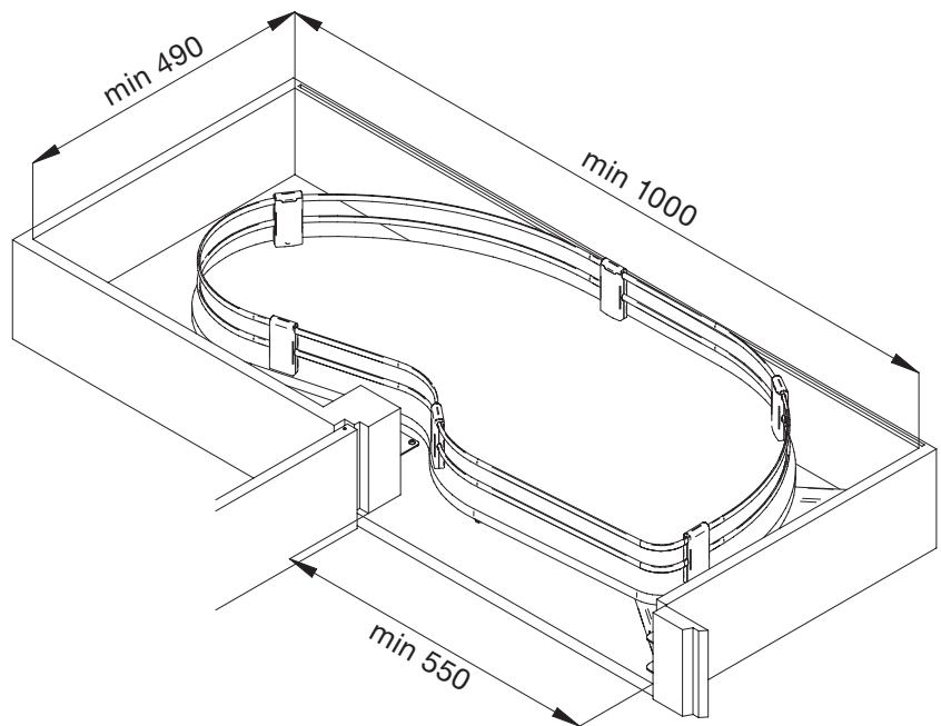
Versione destra Right hand version
